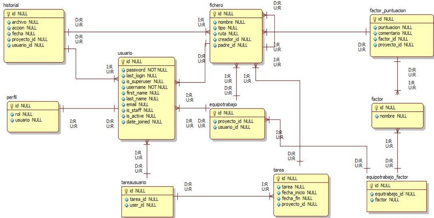
Figura 16 Modelo entidad relación
