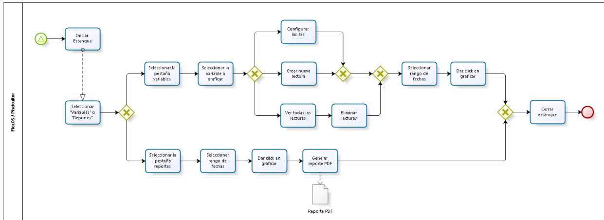
Figura 19. Diagrama de procesos "TO-BE".
