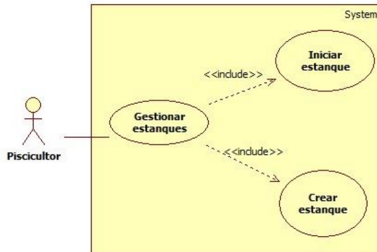
Figura 13. Caso de uso "Gestionar estanques".
