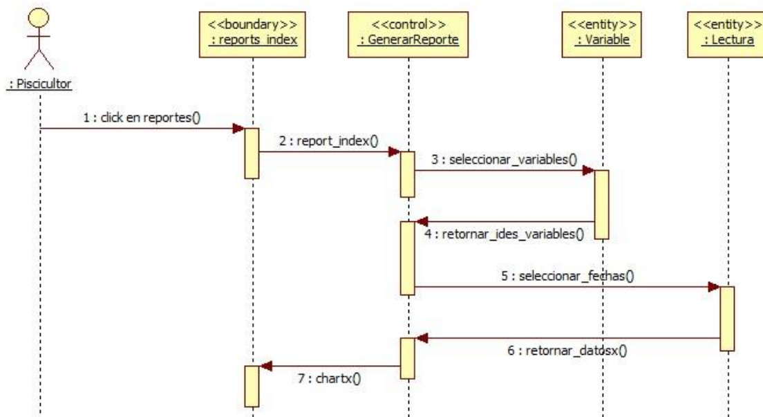
Figura 22. Diagrama de secuencia del CU "Generar reporte".
