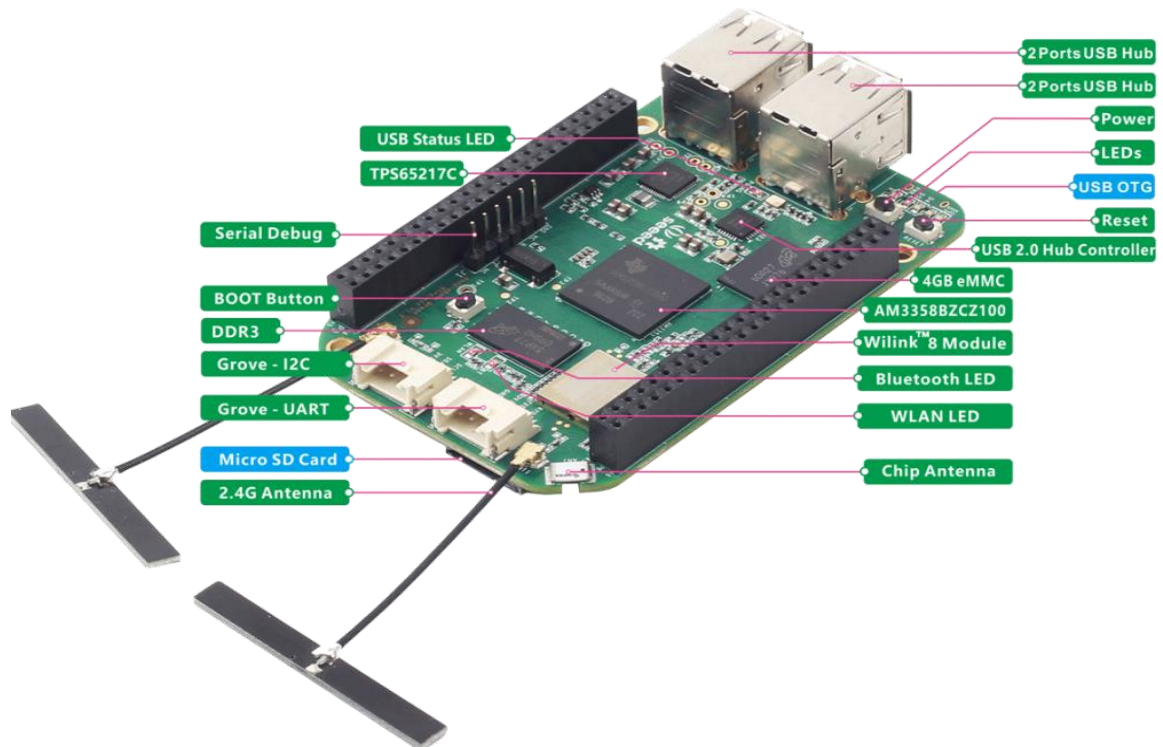
Figura 8. Especificaciones de la BeagleBone Wireless Green
