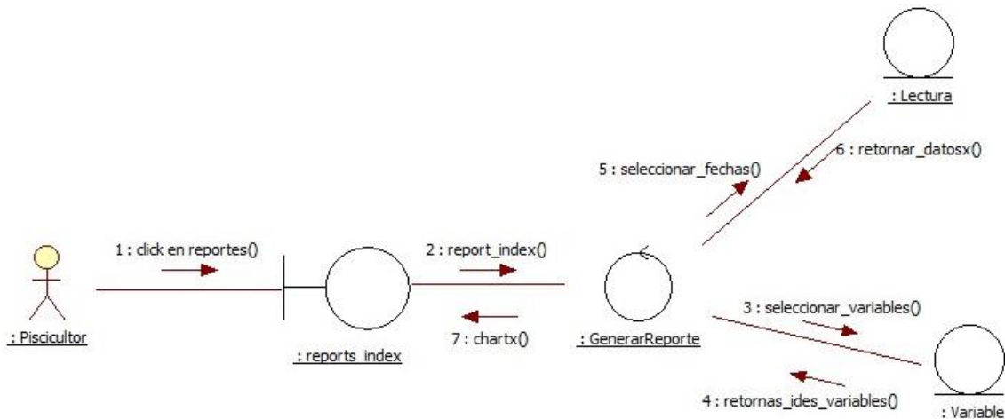
Figura 21. Diagrama de comunicación del CU "Generar reporte".
