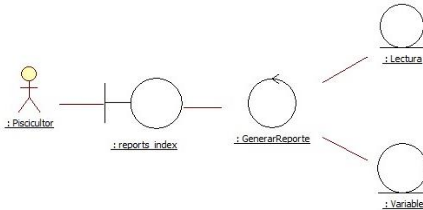
Figura 20 Diagrama de colaboración "Generar reporte".
