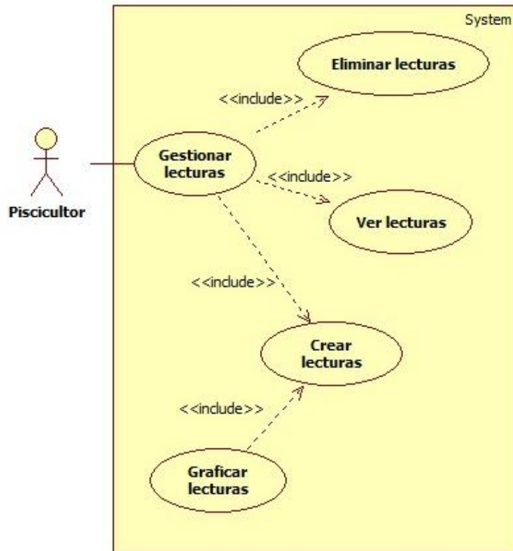
Figura 15. Caso de uso "Gestionar lecturas".
