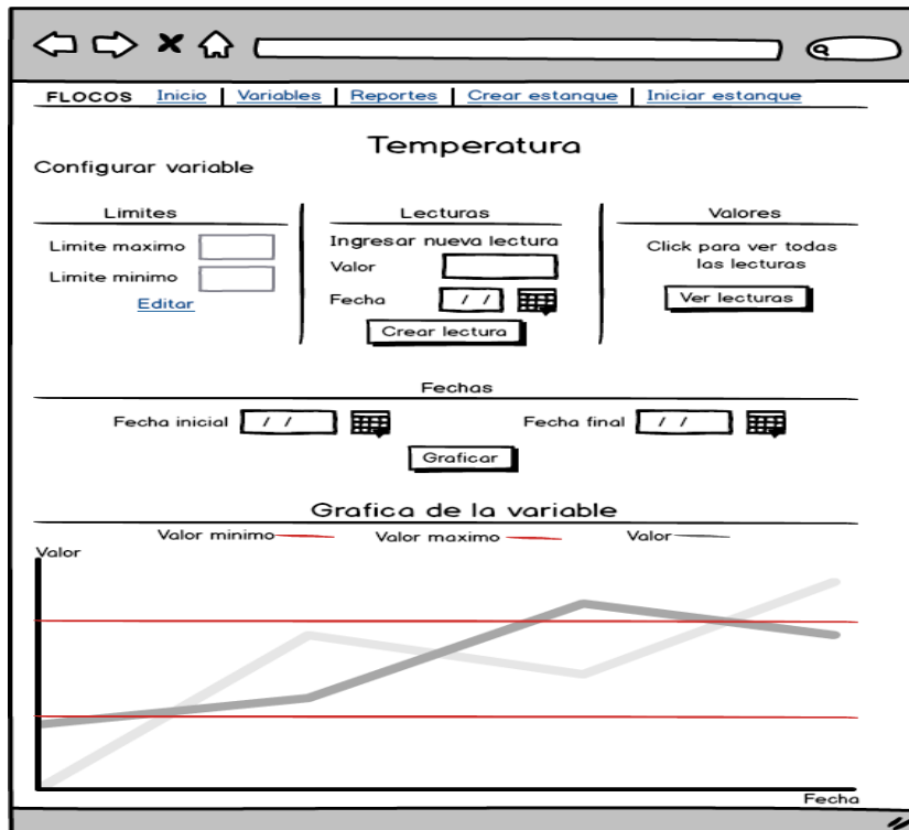
Figura 24. Mockup con varios CU integrados.
