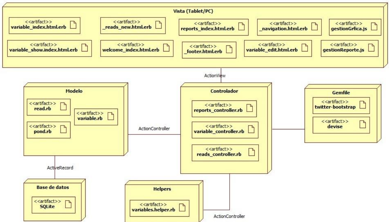
Figura 32. Diagrama de despliegue
