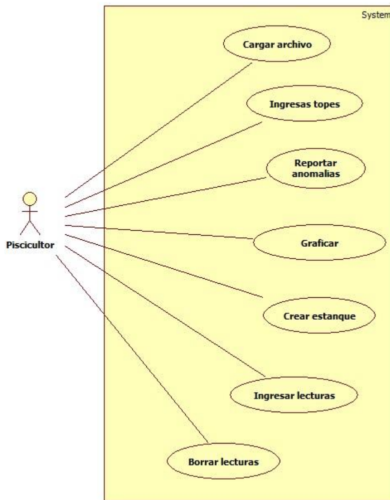
Figura 10. Diagrama de casos de Uso V1.
