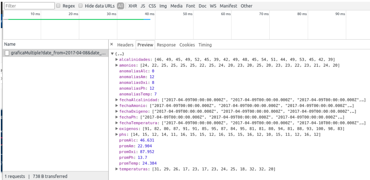
Figura 31. Objeto JSON con los datos del reporte.
