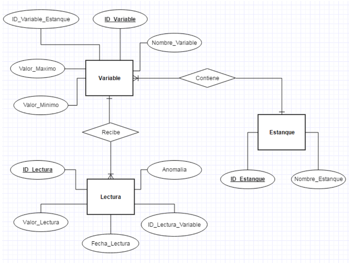
Figura 17. Modelo entidad-relación.
